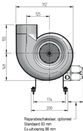
Afb. 1e| Frameuitvoering met DS-Ex-Motor (PPs voor zone 2 | PPs-el voor Zone 1)
