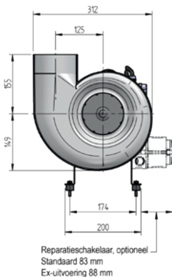
Afb. 1f| Frameuitvoering met WS-Ex-Motor (PPs voor zone 2 | PPs-el voor Zone 1)
