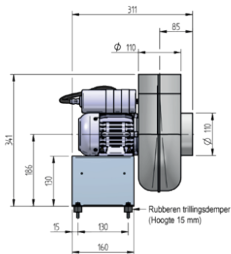
Afb. 1e| Frameuitvoering met DS-Ex-Motor (PPs voor zone 2 | PPs-el voor Zone 1)
